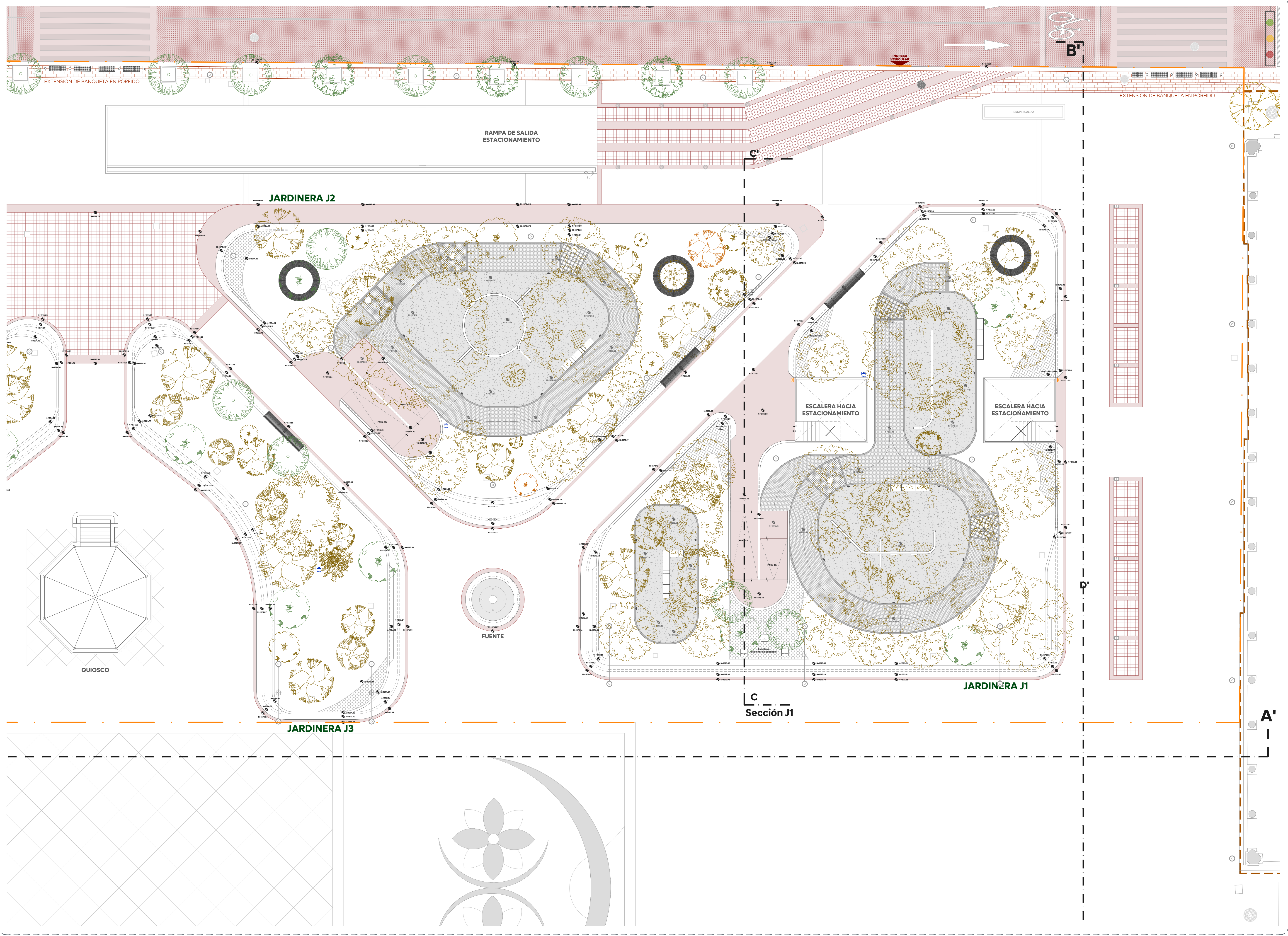
01 Planta Arquitectónica Primer Cuadrante 1:125
