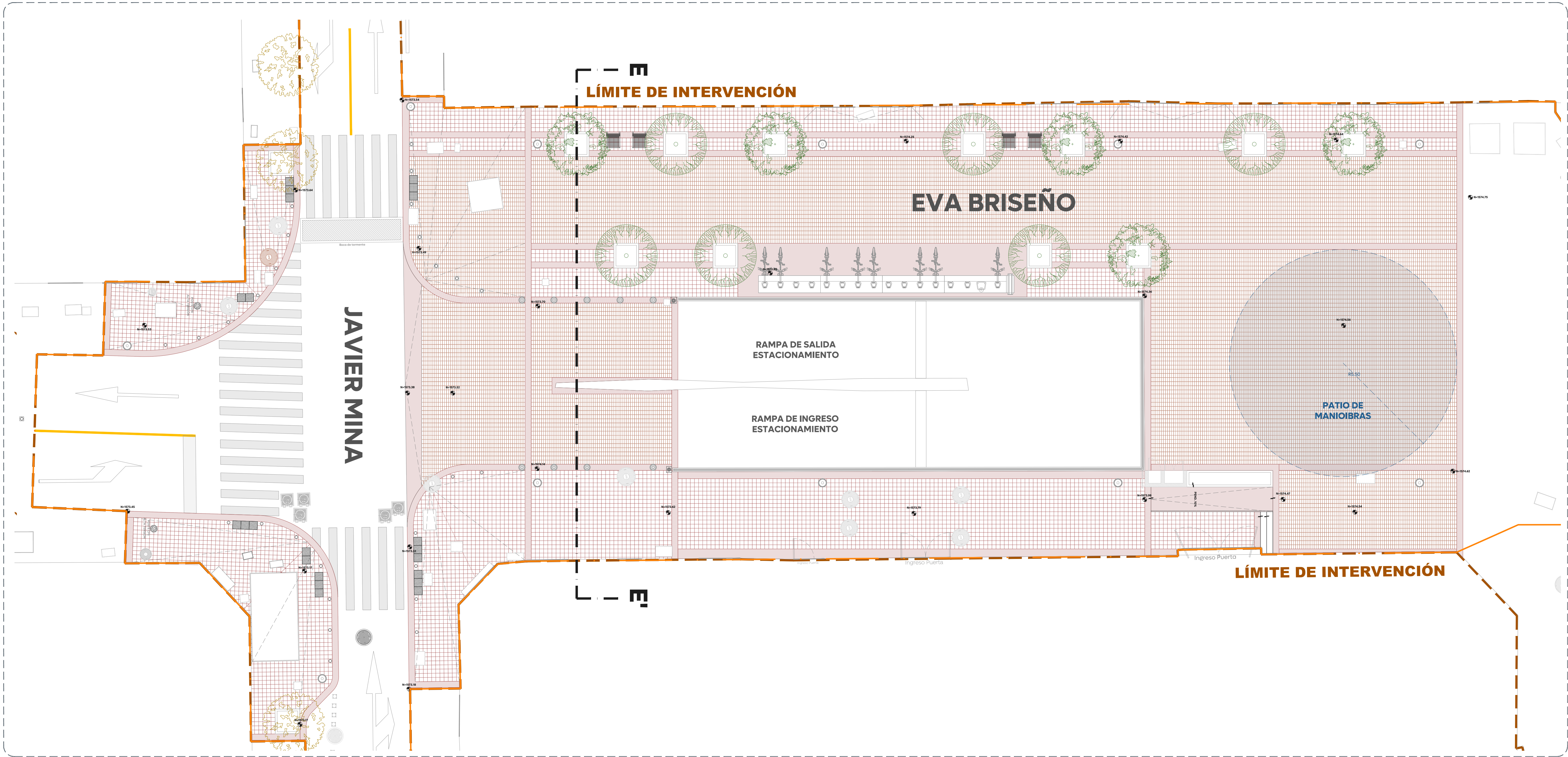
01 Planta arquitectónica Andador Eva Briseño 1:100
