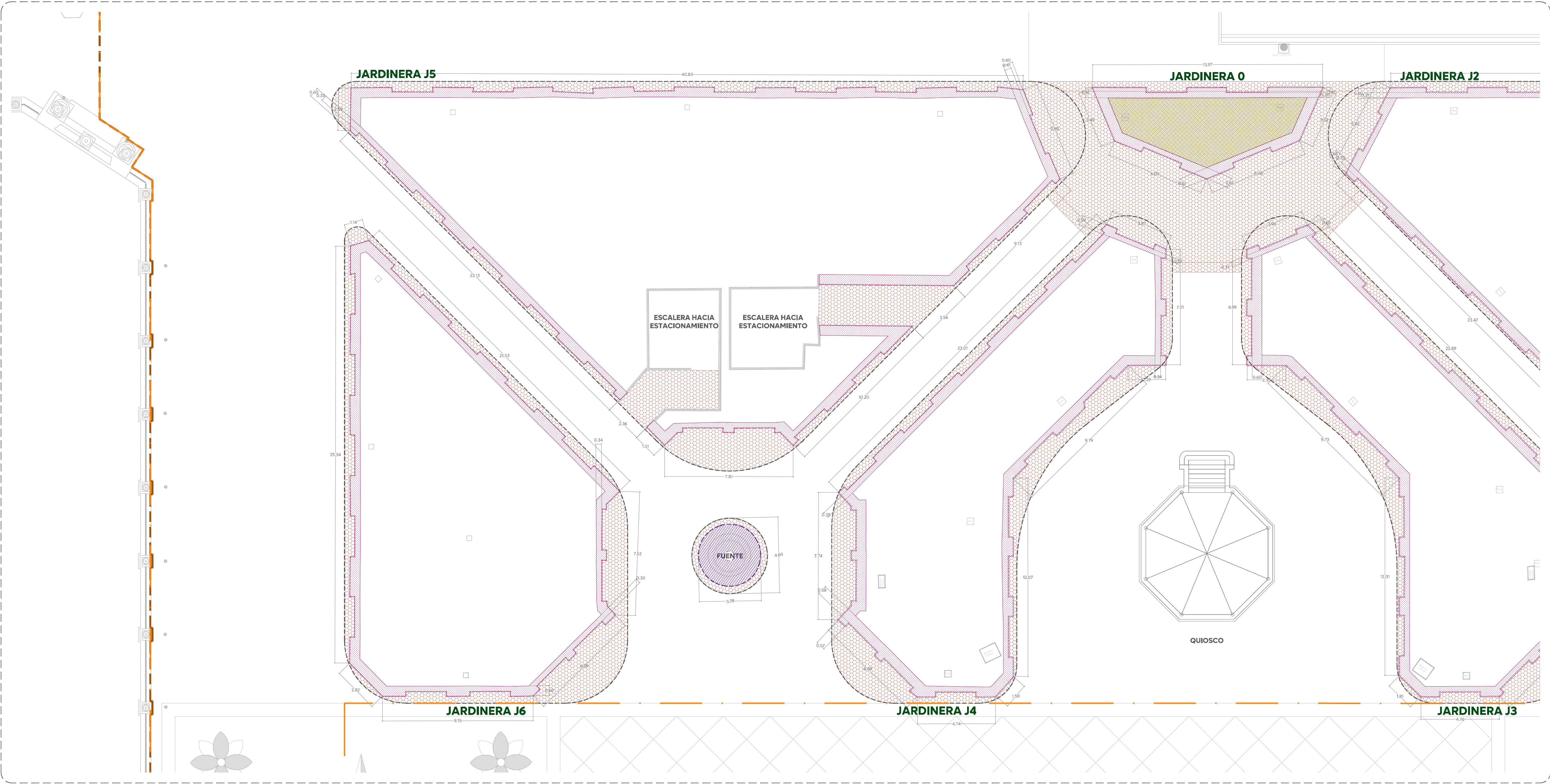
01 Planta de Demoliciones Tercer Cuadrante 1:125
