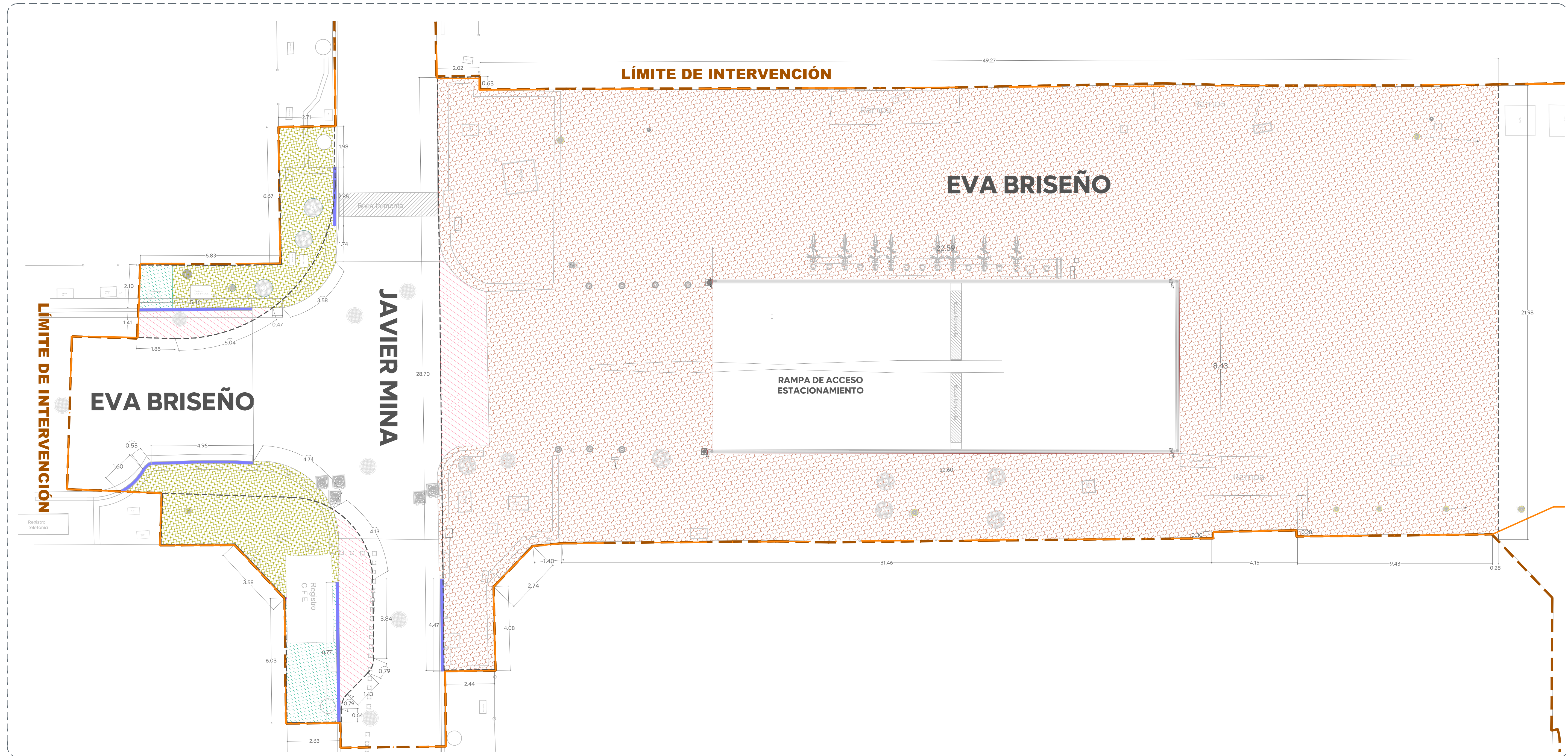
01 Planta de Demoliciones Andador Eva Briseño 1:100
