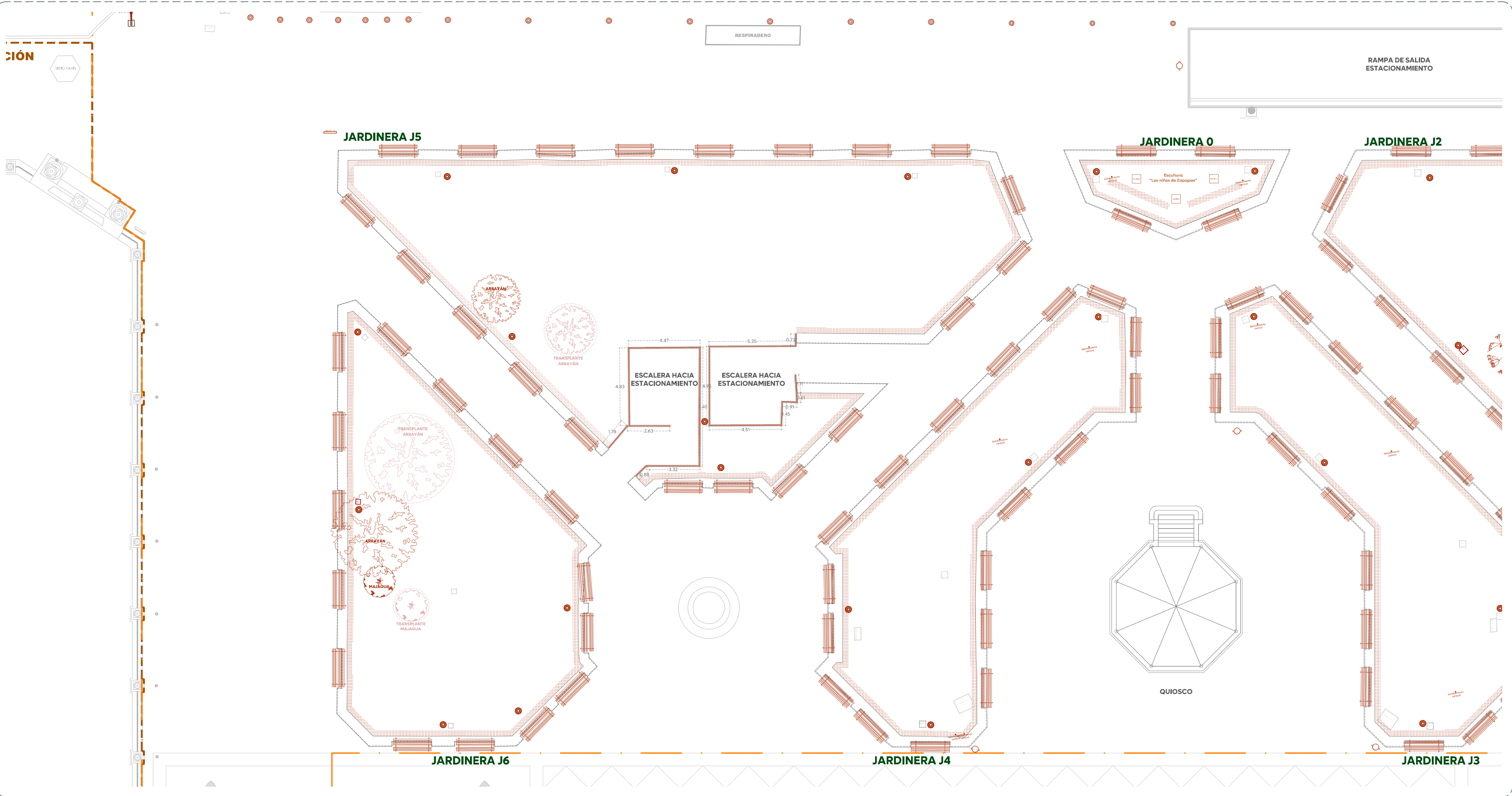
01 Planta de Retiros Tercer Cuadrante 1:125
