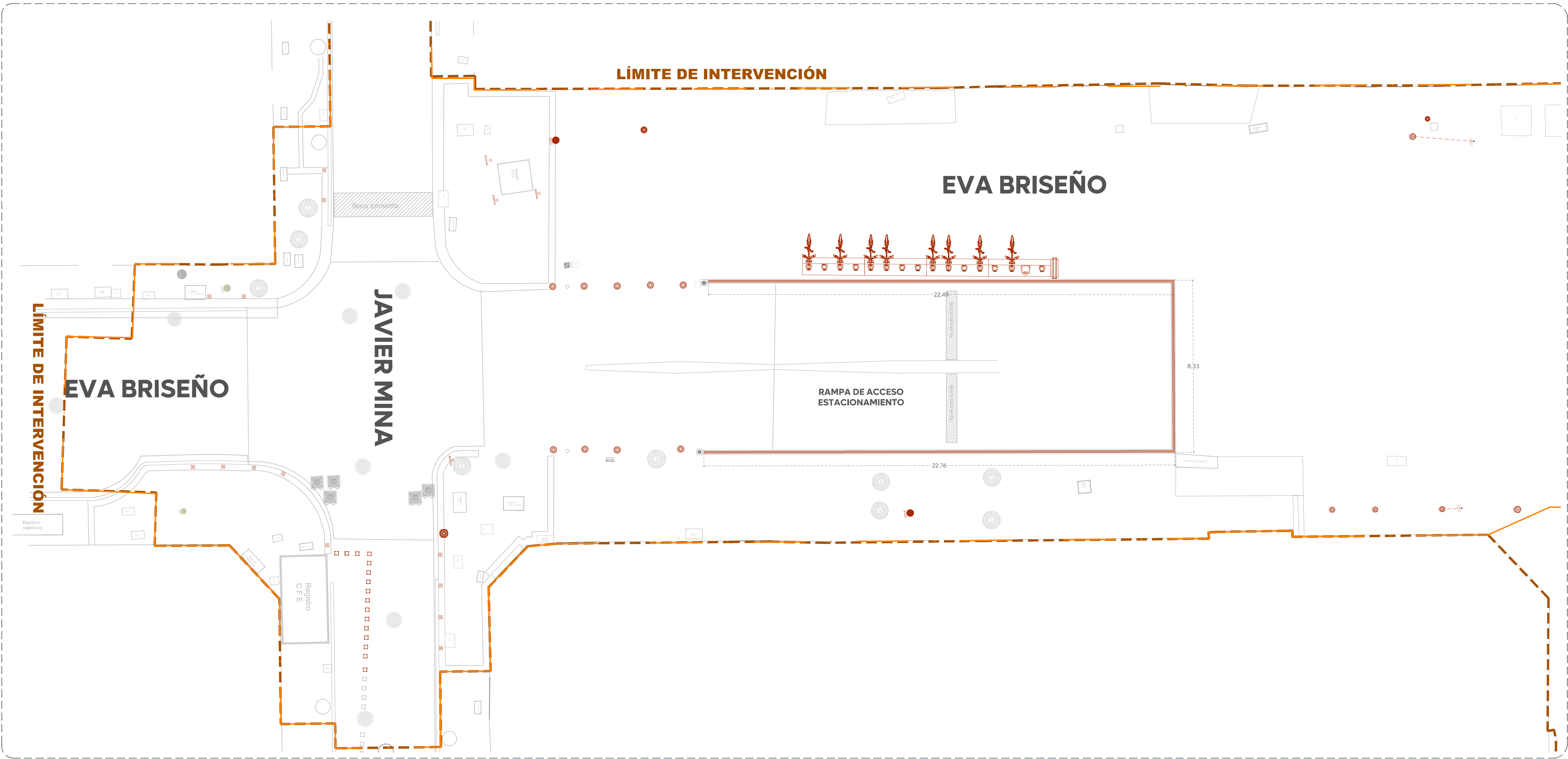
01 Planta de Retiros Andador Eva Briseño 1:100
