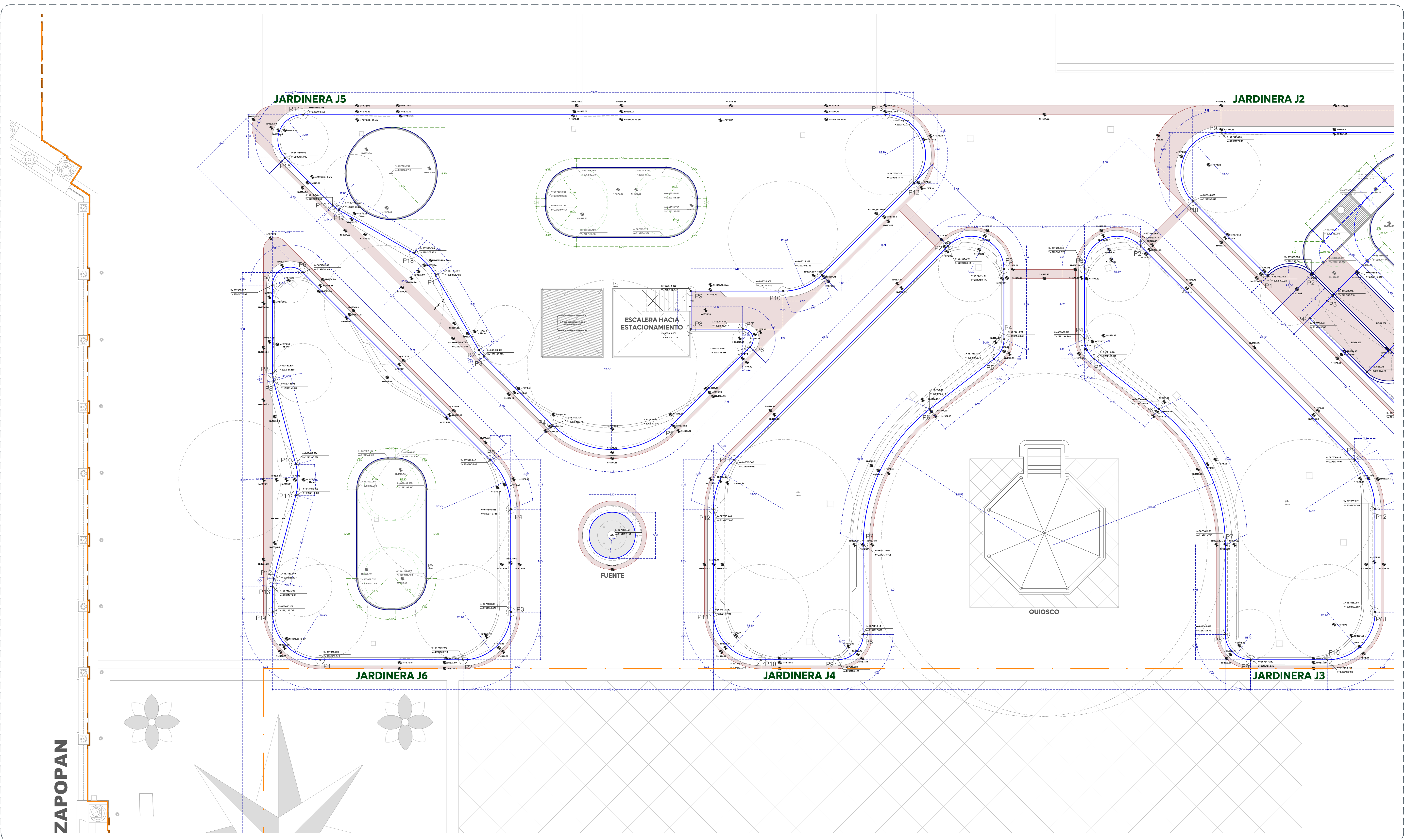
01 Planta de Trazo Tercer Cuadrante 1:125
