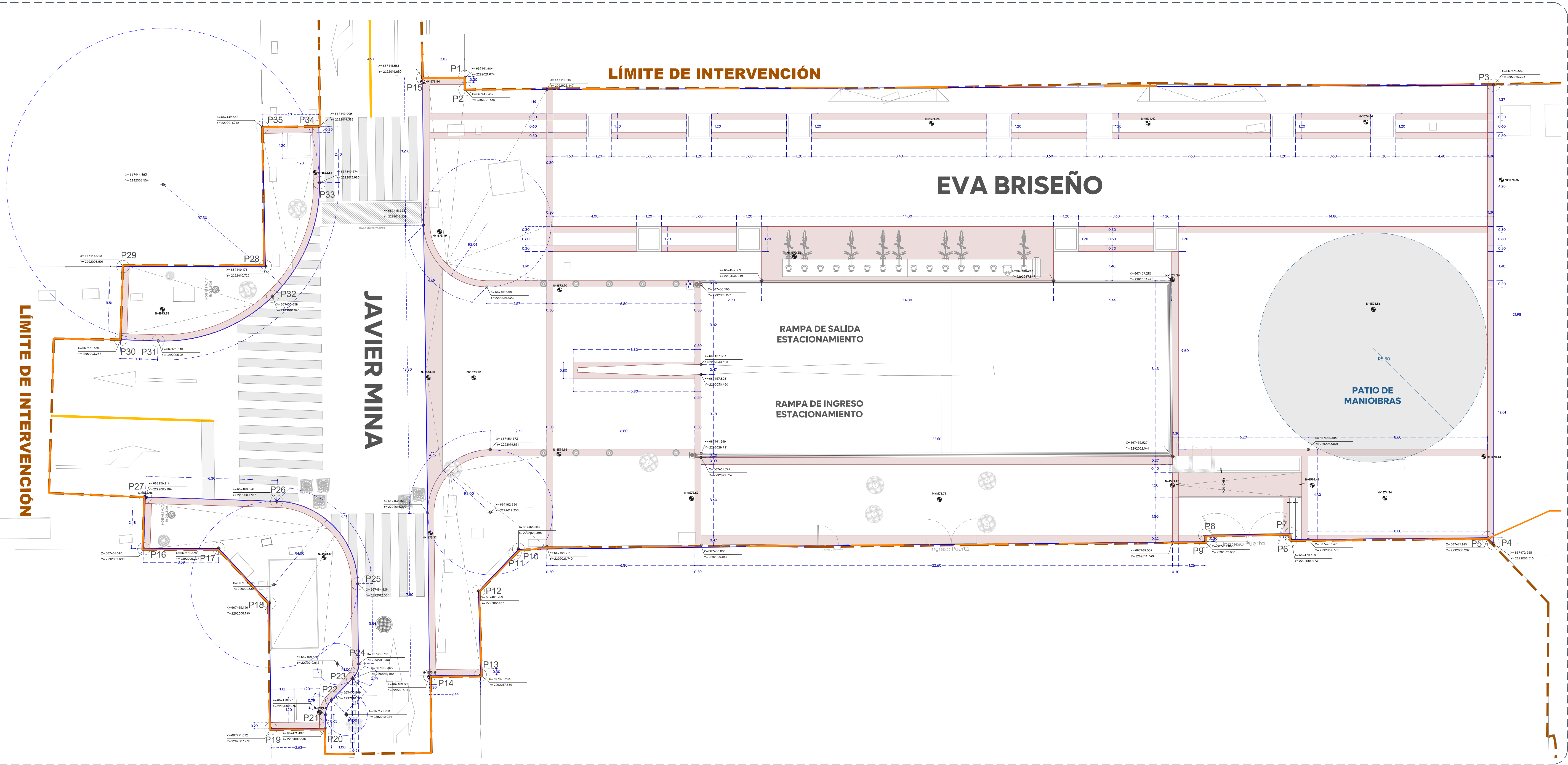
01 Planta de Trazo Andador Eva Briseño 1:100
