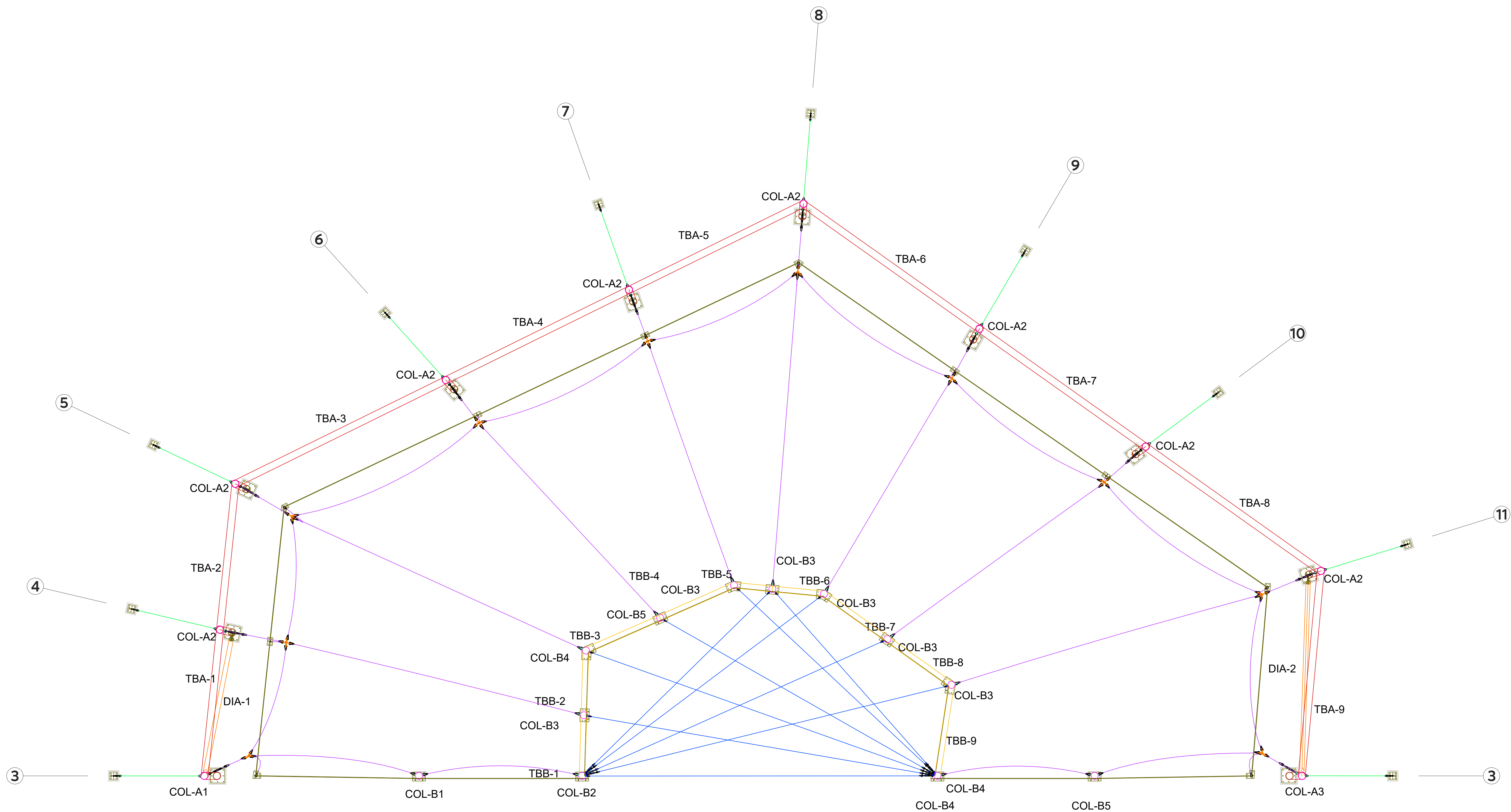
02 Planta de Elementos Estructurales Hábitat de felinos Esc. 1:100
