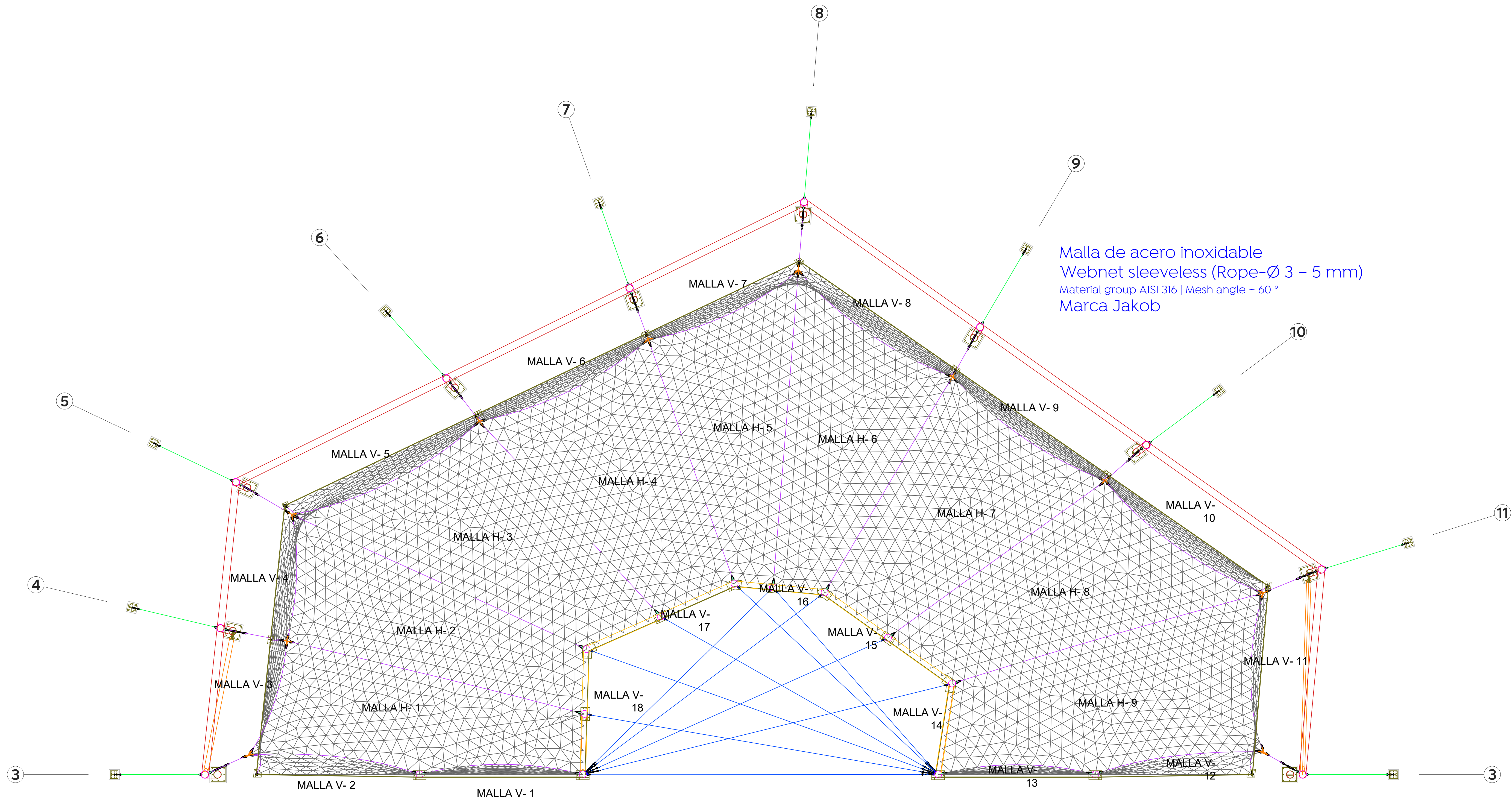
04 Planta de Mallas Hábitat de felinos Esc. 1:100
