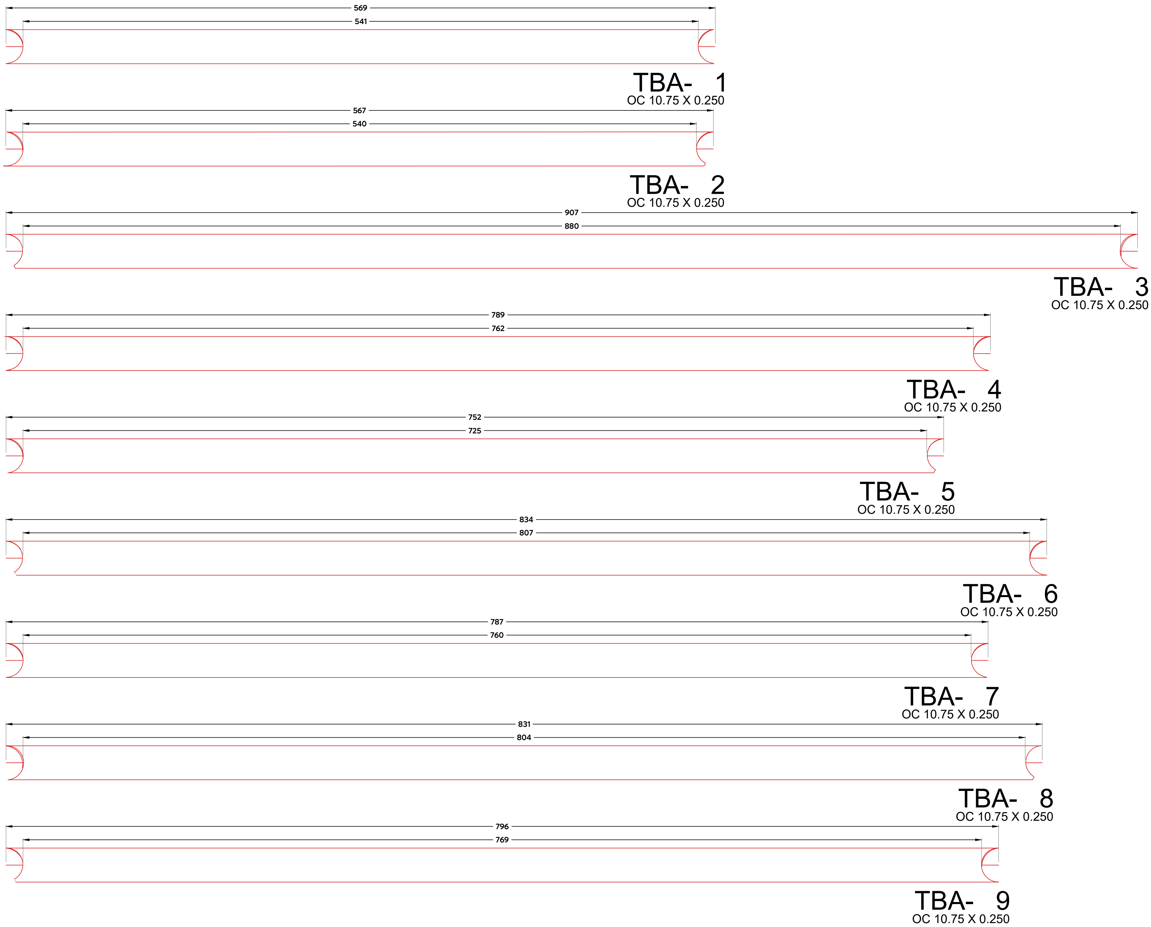
15 TRABES TIPO A Hábitat de felinos Esc. 1:100
