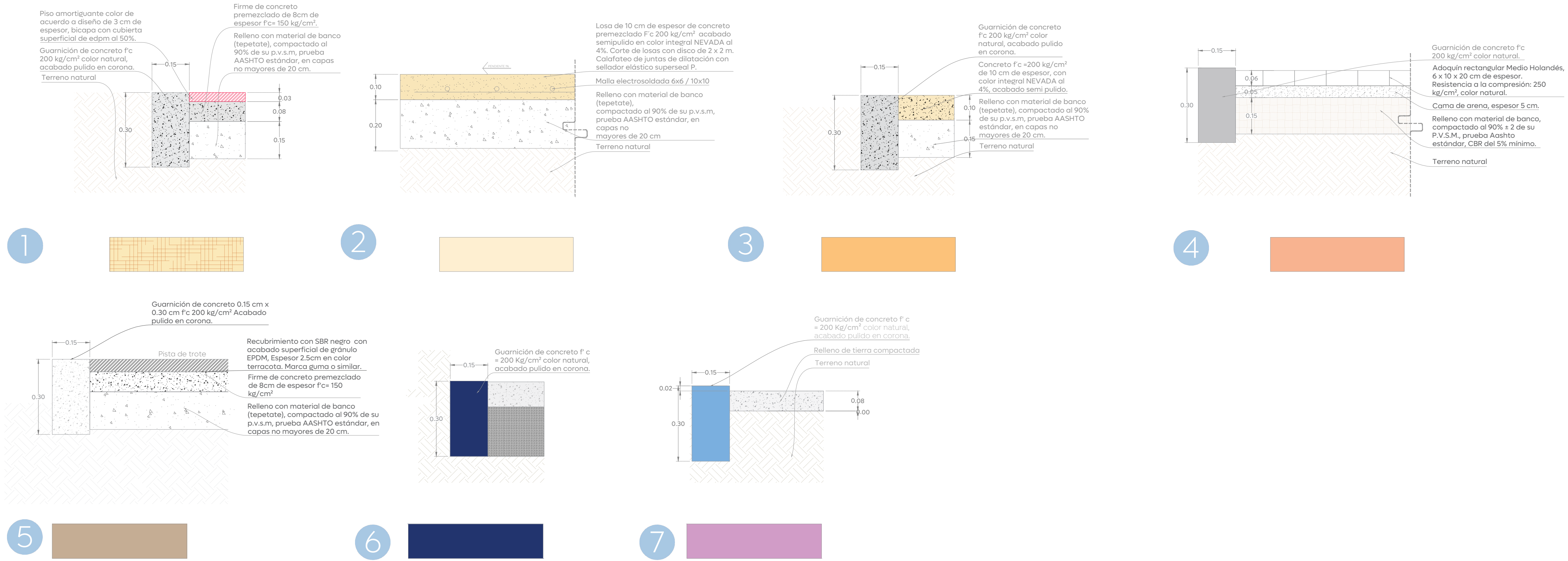
02 Detalle de acabados en piso Acabados 1:10
