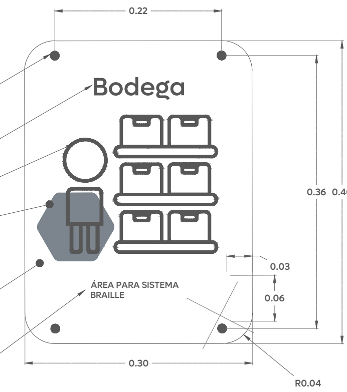
04 DT-SÑ-01 Detalle tipo de módulos de señalética Esc. 1:5
