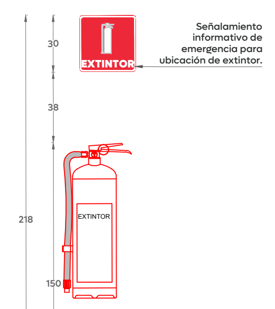
05 DT-SÑ-02 Montaje en Muro Esc. 1:30
