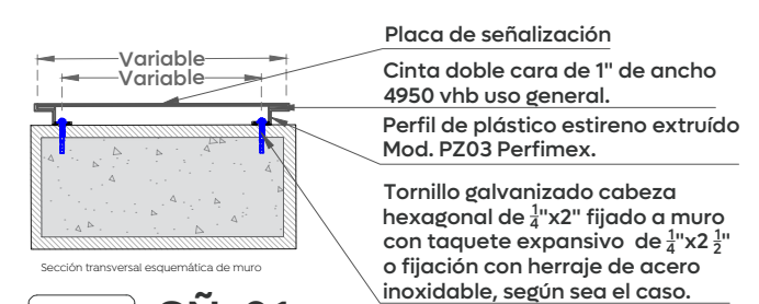
06 SÑ-01 Fijación en superficies irregulares Esc. 1:10
