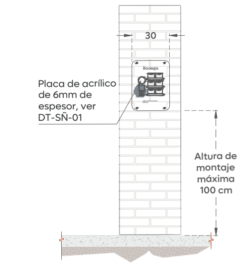
05 DT-SÑ-02 Montaje en Muro Esc. 1:30
