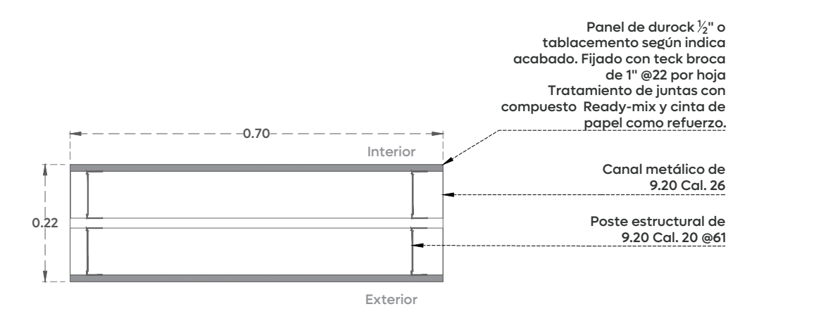
01 AL-05 Muro de tablaroca de 22 cm Esc. 1:10
