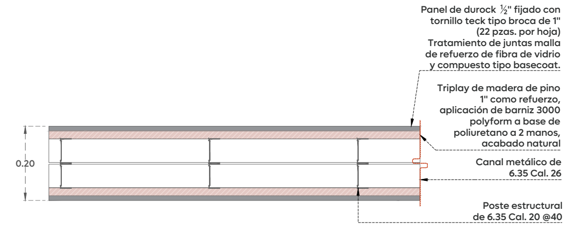
01 AL-06 Muro de tablaroca de 20 cm Esc. 1:10
