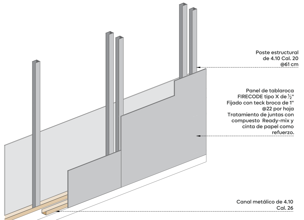
01 AL-03 Muro de tablaroca de 20 cm Esc. 1:10
