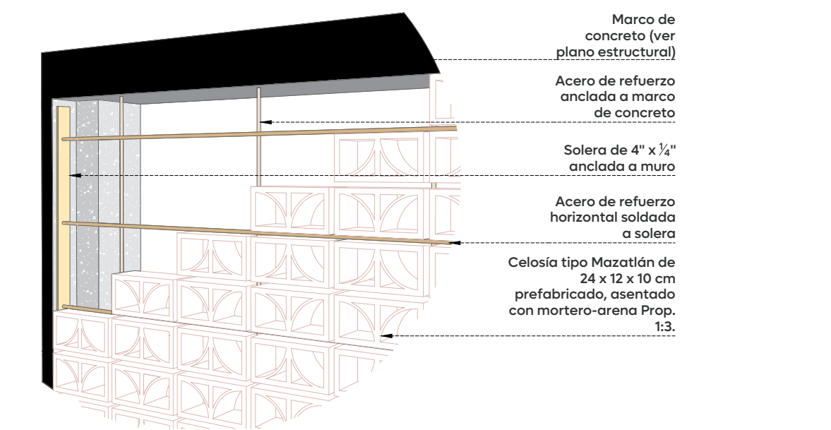
01 AL-01 Detalle muro de celosía Esc. 1:20
