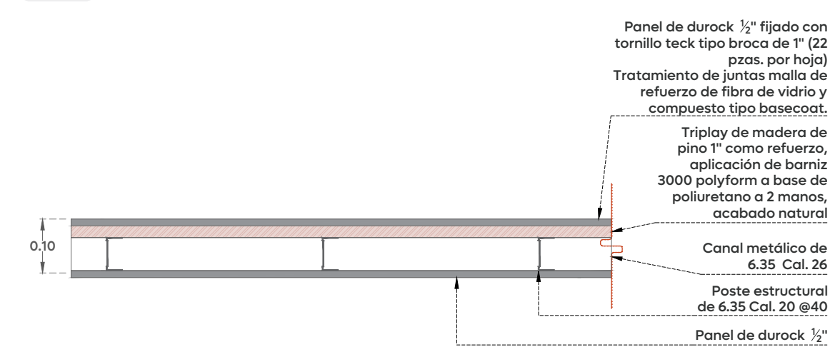
01 AL-07 Muro de tablaroca de 10 cm Esc. 1:10
