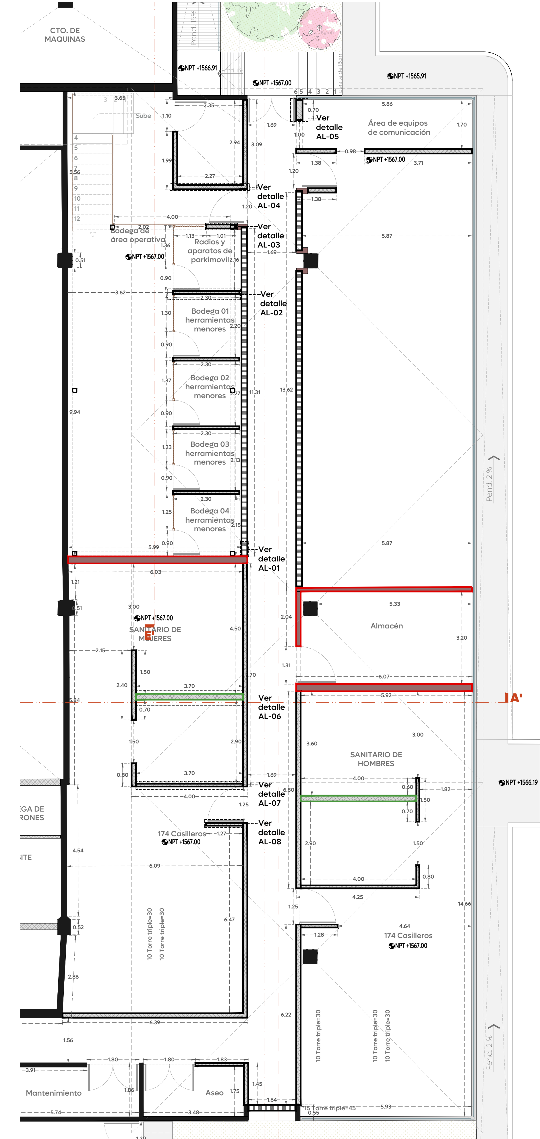
01 Planta Muros Dirección de Movilidad y Tránsito de Zapopan. Esc. 1:75
