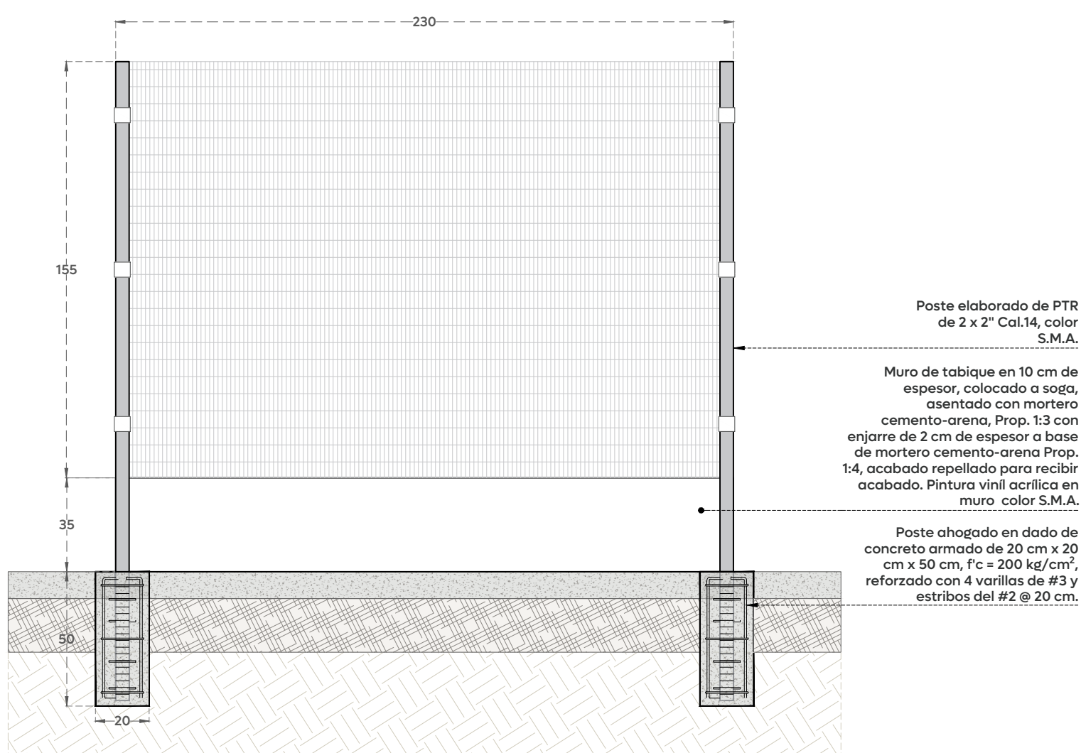
01 AL-02 Detalle muro bajo de tabique Esc. 1:20
