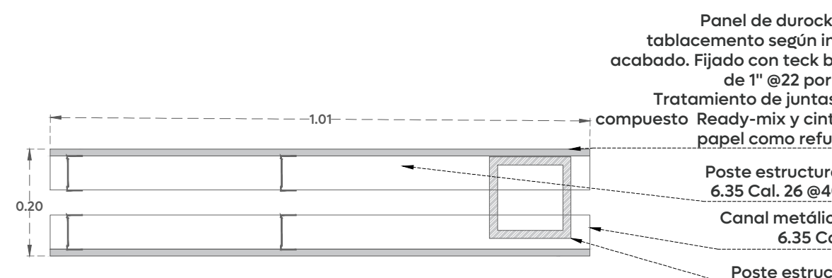
01 AL-03 Muro de tablaroca de 20 cm Esc. 1:10
