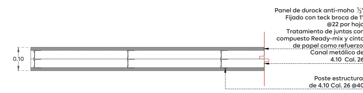
01 AL-08 Muro de tablaroca de 10 cm Esc. 1:10
