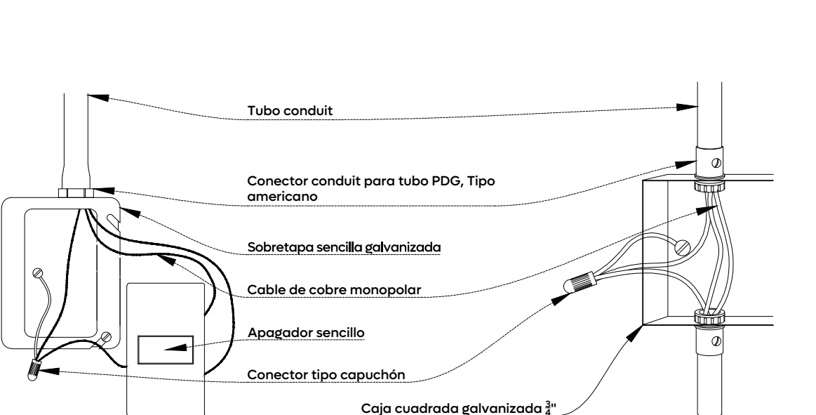
05 Detalle típico de apagador sencillo IE-03 S/E
