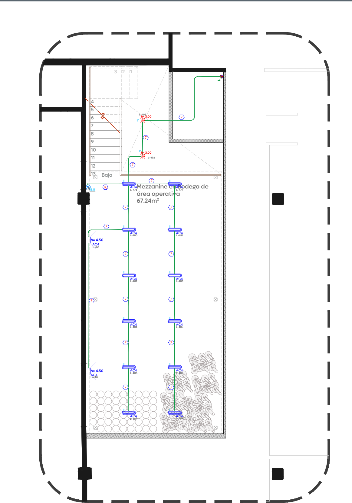
02 Planta iluminación mezzanine IE-03 Esc. 1:100
