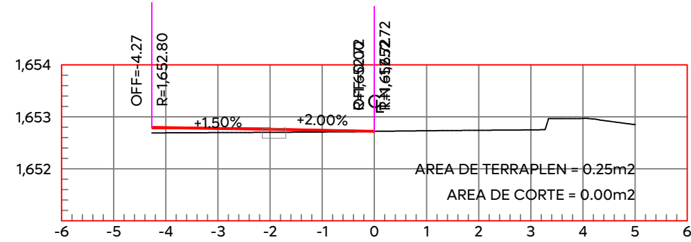
ESTACION 0+294.46 ESCALA HORIZONTAL 1:100 ESCALA VERTICAL 1:100
