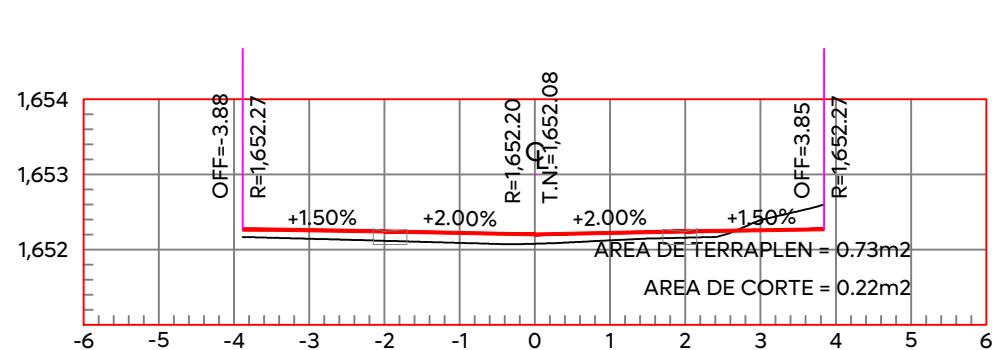
ESTACION 0+180.00 ESCALA HORIZONTAL 1:100 ESCALA VERTICAL 1:100
