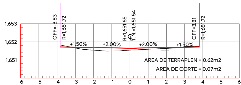
ESTACION 0+080.00 ESCALA HORIZONTAL 1:100 ESCALA VERTICAL 1:100
