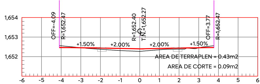
ESTACION 0+220.00 ESCALA HORIZONTAL 1:100 ESCALA VERTICAL 1:100
