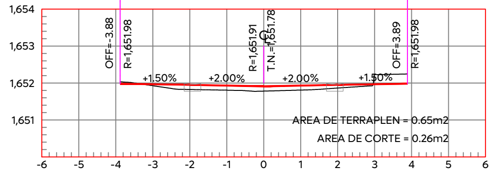
ESTACION 0+120.00 ESCALA HORIZONTAL 1:100 ESCALA VERTICAL 1:100
