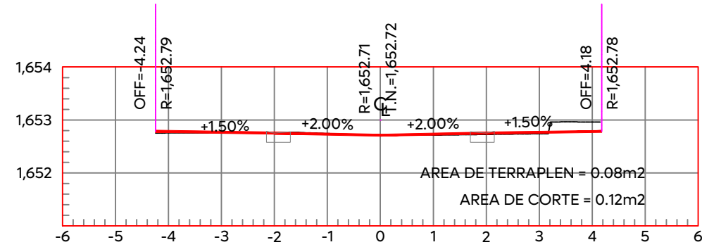
ESTACION 0+291.80 ESCALA HORIZONTAL 1:100 ESCALA VERTICAL 1:100
