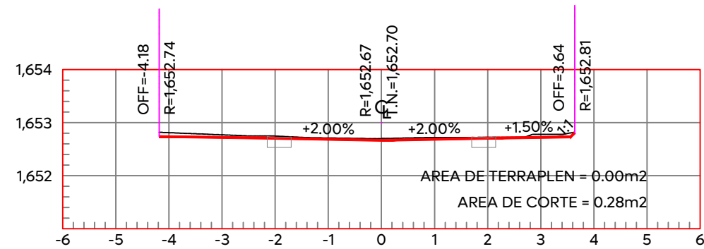
ESTACION 0+280.00 ESCALA HORIZONTAL 1:100 ESCALA VERTICAL 1:100
