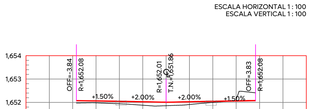
ESTACION 0+140.00 ESCALA HORIZONTAL 1:100 ESCALA VERTICAL 1:100
