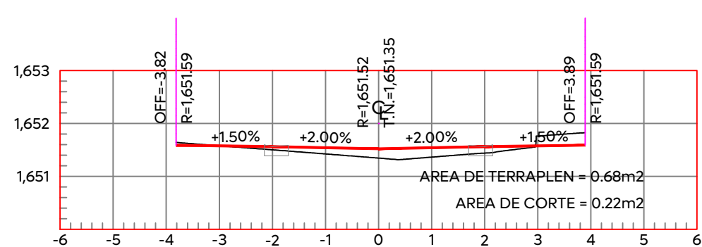
ESTACION 0+060.00 ESCALA HORIZONTAL 1:100 ESCALA VERTICAL 1:100
