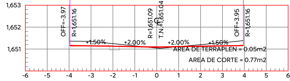
ESTACION 0+020.00 ESCALA HORIZONTAL 1:100 ESCALA VERTICAL 1:100
