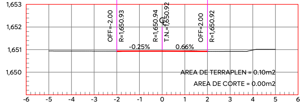
ESTACION 0+008.25 ESCALA HORIZONTAL 1:100 ESCALA VERTICAL 1:100
