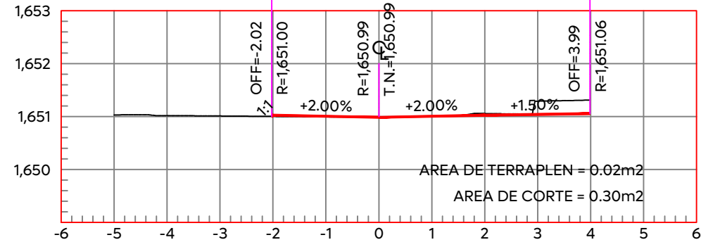
ESTACION 0+013.31 ESCALA HORIZONTAL 1:100 ESCALA VERTICAL 1:100
