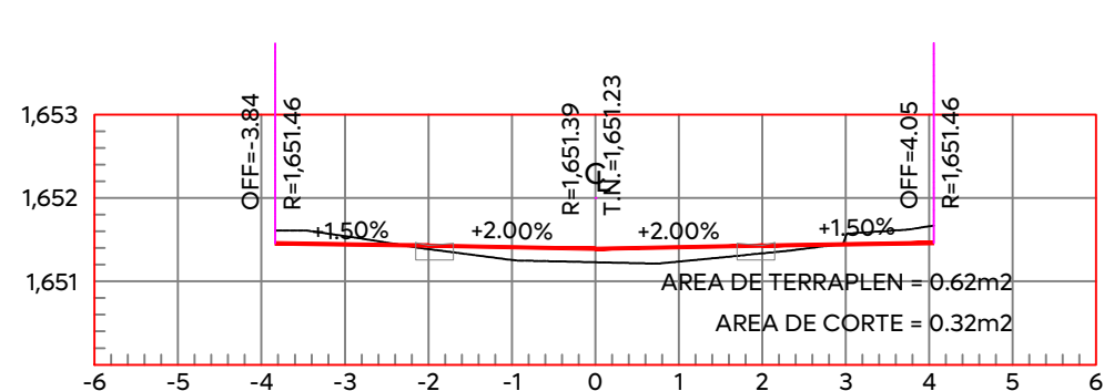
ESTACION 0+040.00 ESCALA HORIZONTAL 1:100 ESCALA VERTICAL 1:100
