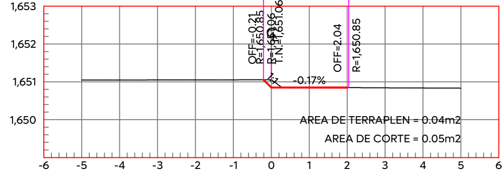
ESTACION 0+000.00 ESCALA HORIZONTAL 1:100 ESCALA VERTICAL 1:100
