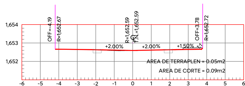
ESTACION 0+260.00 ESCALA HORIZONTAL 1:100 ESCALA VERTICAL 1:100
