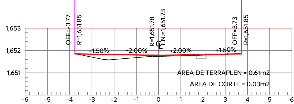
ESTACION 0+100.00 ESCALA HORIZONTAL 1:100 ESCALA VERTICAL 1:100
