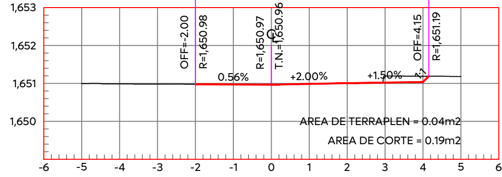
ESTACION 0+011.36 ESCALA HORIZONTAL 1:100 ESCALA VERTICAL 1:100
