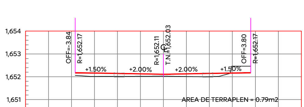
ESTACION 0+160.00 ESCALA HORIZONTAL 1:100 ESCALA VERTICAL 1:100
