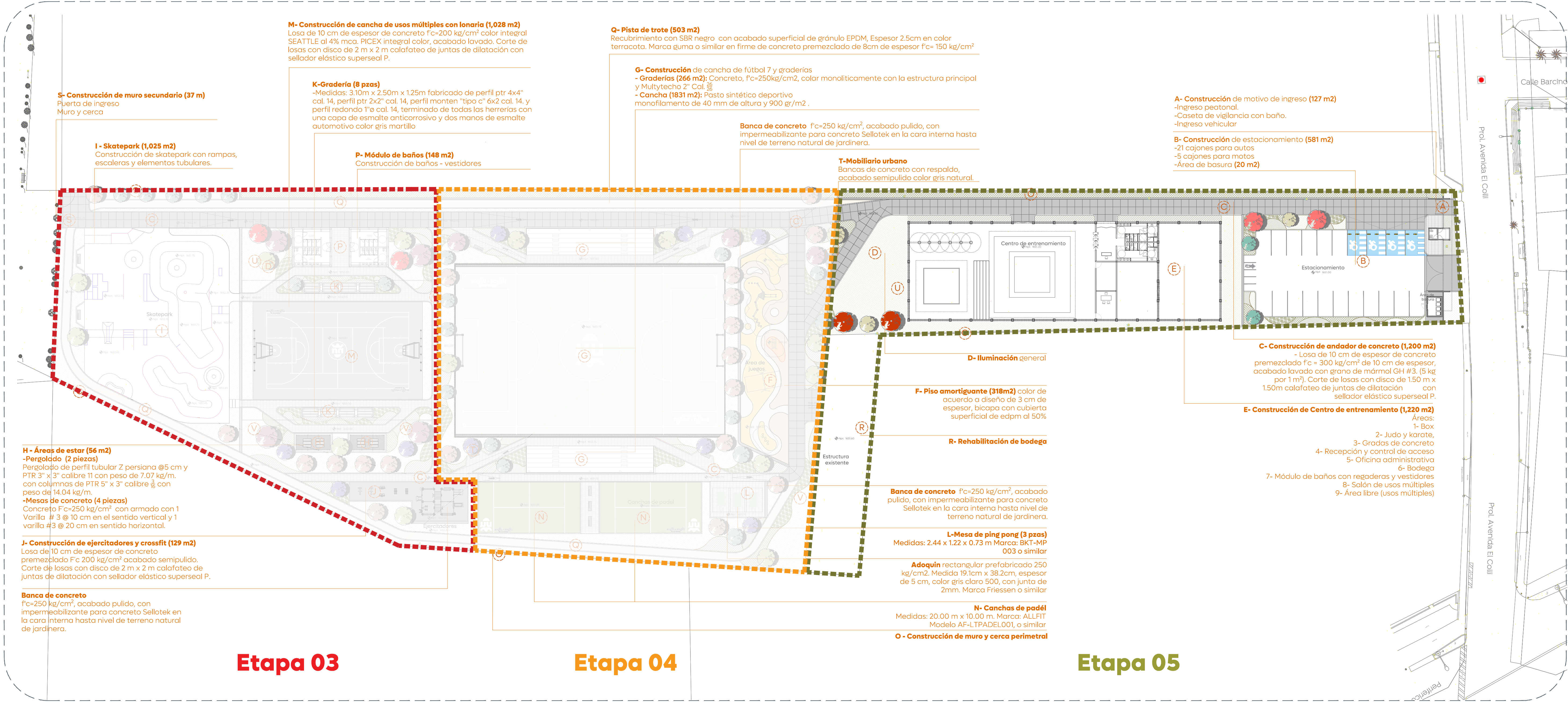
01 Plano llave Arquitectónico y Alcances Generales 1:400
